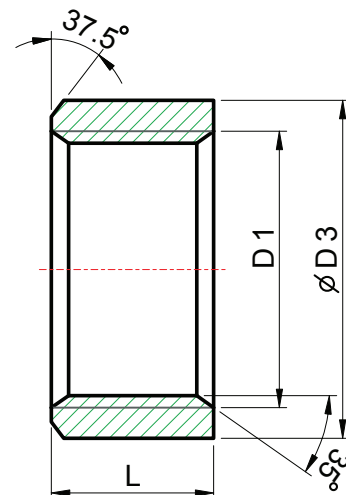
BSP, DIN2999
